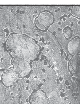
ALH 84001 ലെ തന്മാത്രാ കണങ്ങളുടെ മൈക്രോസ്കോപ്പ് ദൃശ്യം
